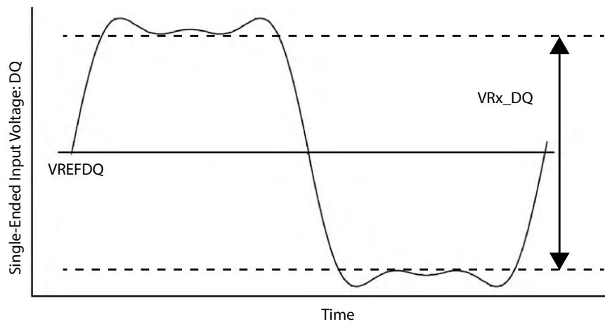
Figure 233 — VRx_DQ
